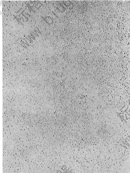
Dense
